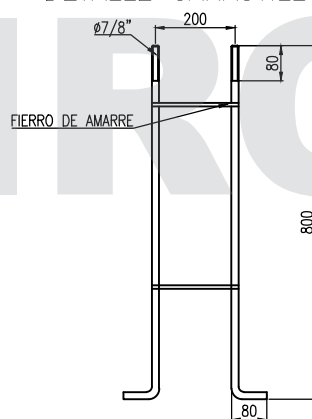
DETALLE CANASTILLO
