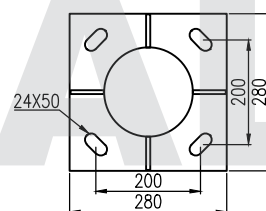
DETALLE PLACA
